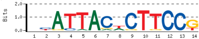
primary_MA0062_MA0094
