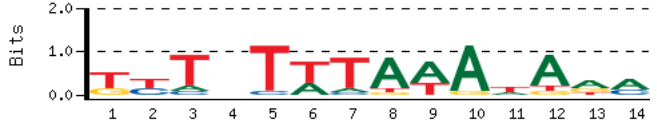
primary_MA0052_MA0053_trimmed
